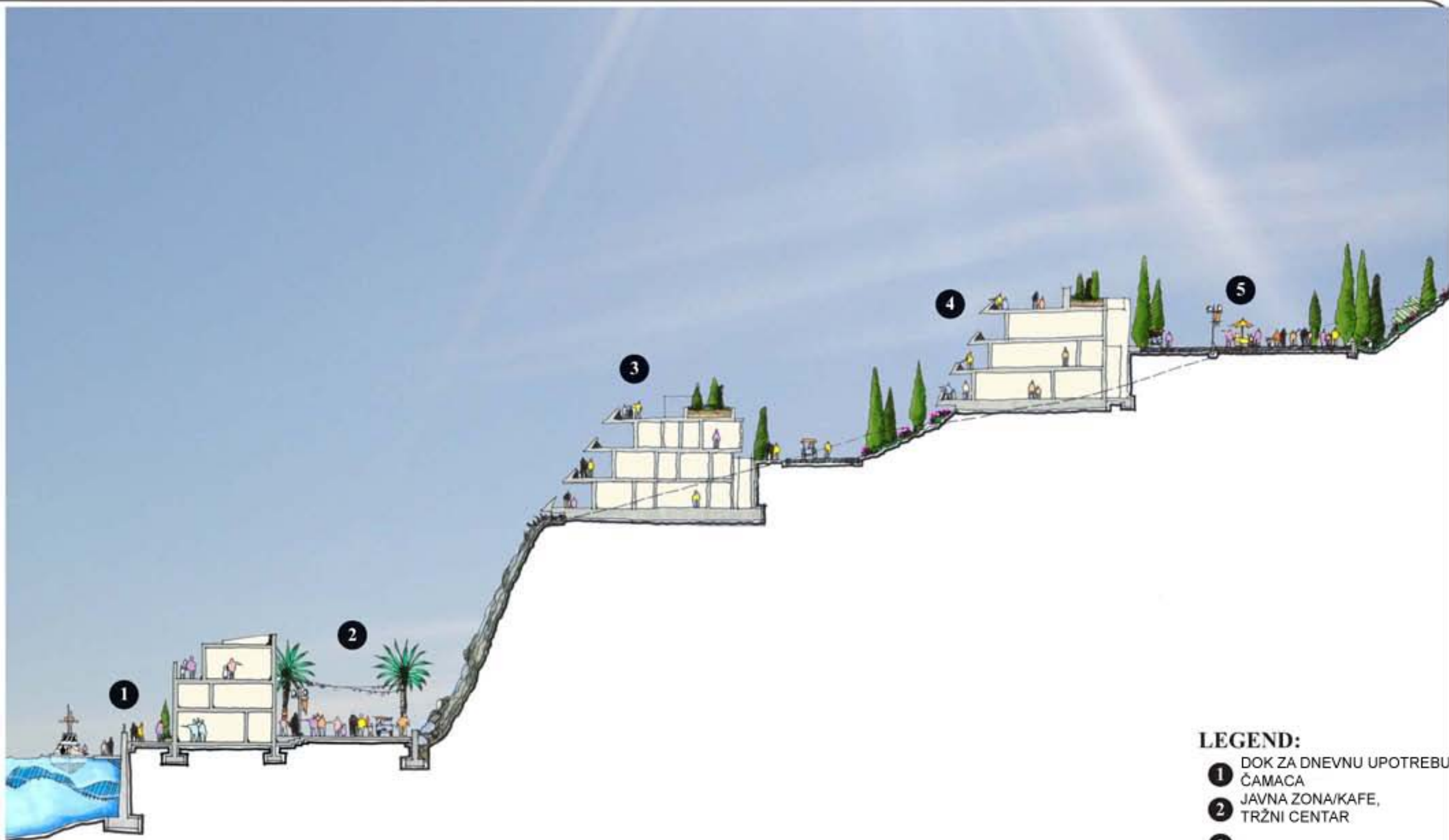
© PRESJEK KROZ VILE I ZONU SA JAVNIM SADRŽAJIMA R/ 1:200
