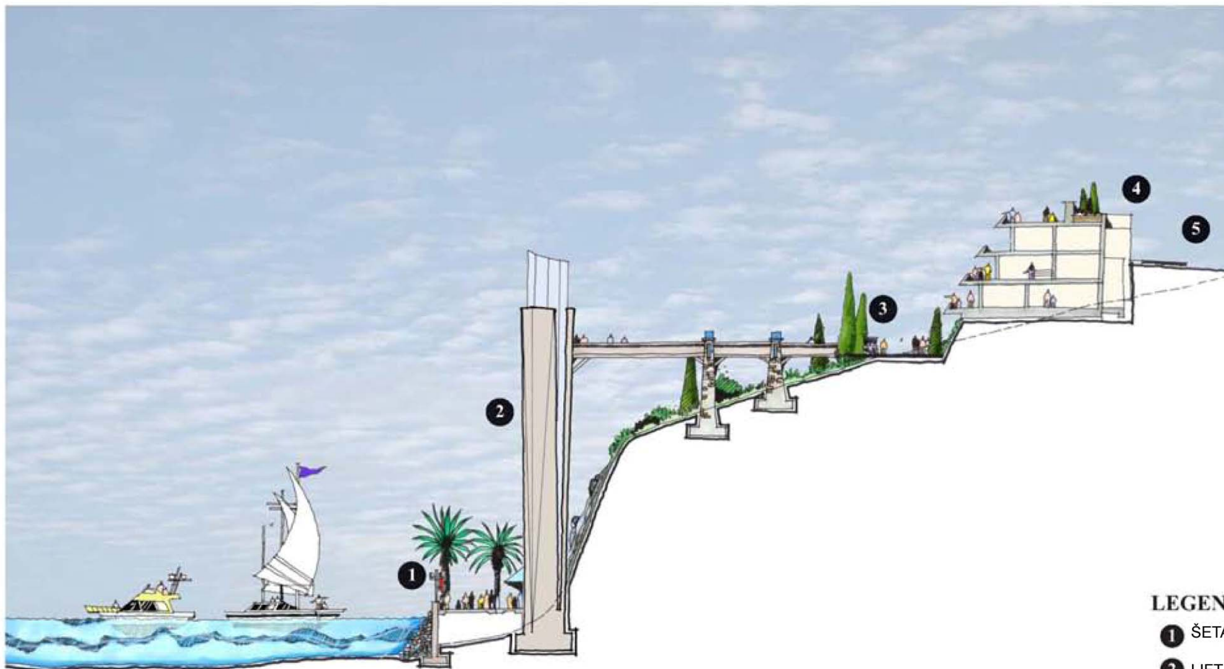
B PRESJEK KROZ PANORAMSKI LIFT I ŠETALIŠTE R/ 1:200
