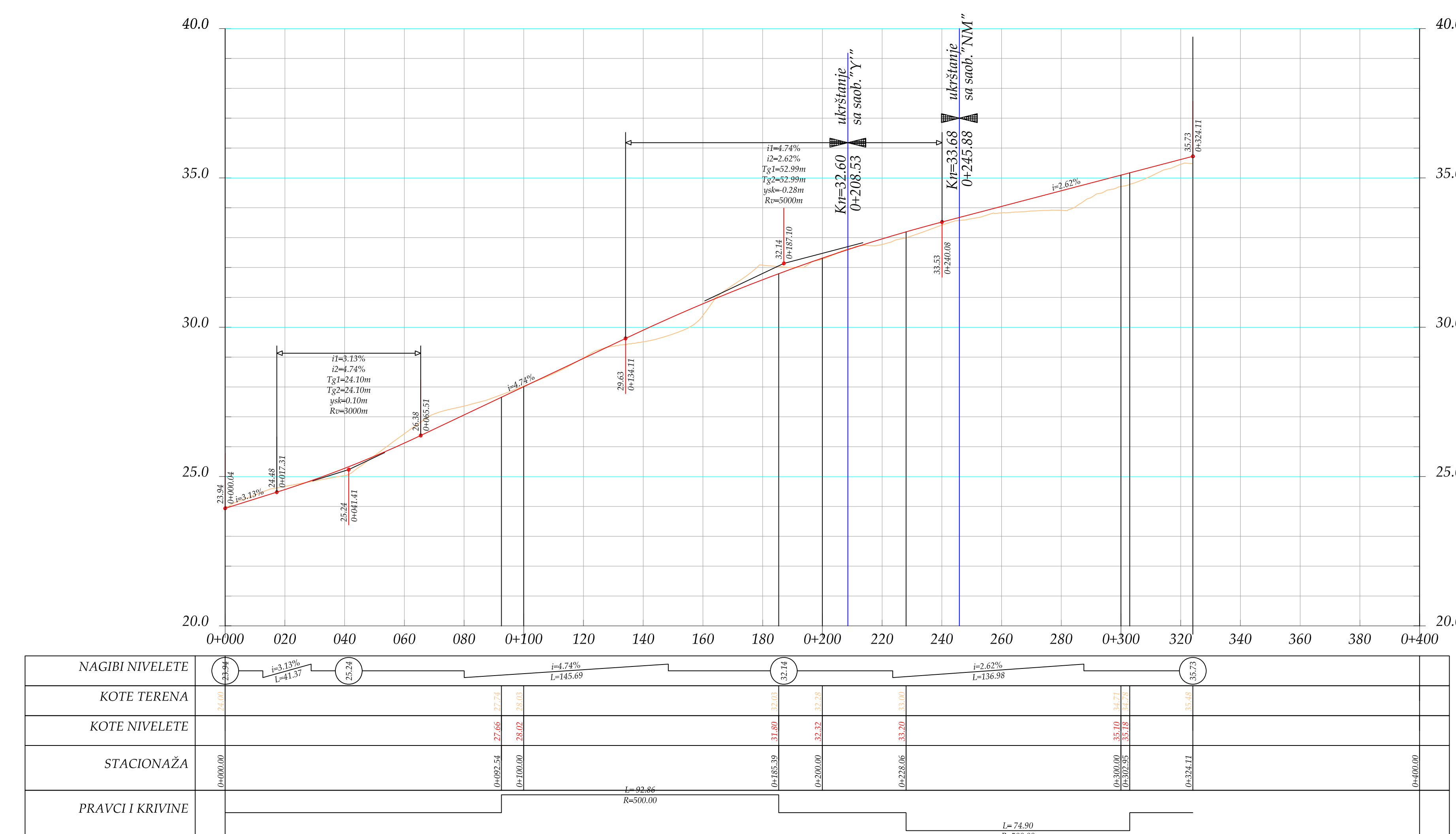
8. UZDUŽNI PROFIL SAOBRAĆAJNICE "X" R 1:100/1000
