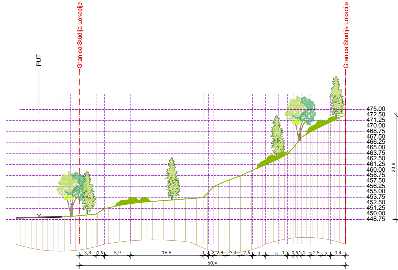
PRESJEK 1-1
