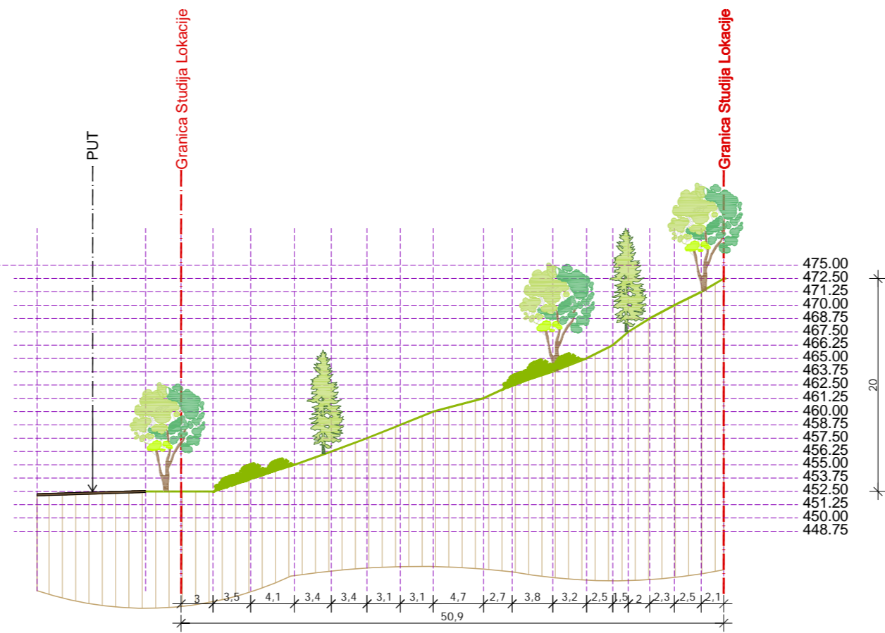
PRESJEK 2-2
