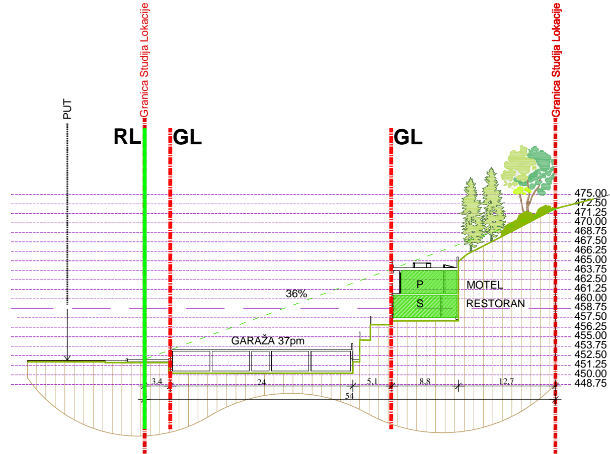
PRESJEK 2-2
