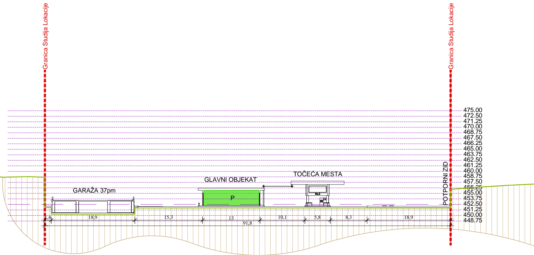
PRESJEK 2-2
