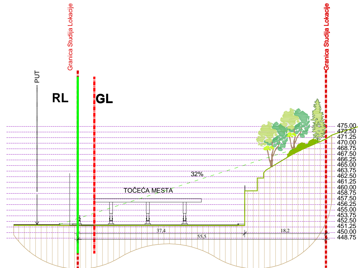
PRESJEK 4-4
