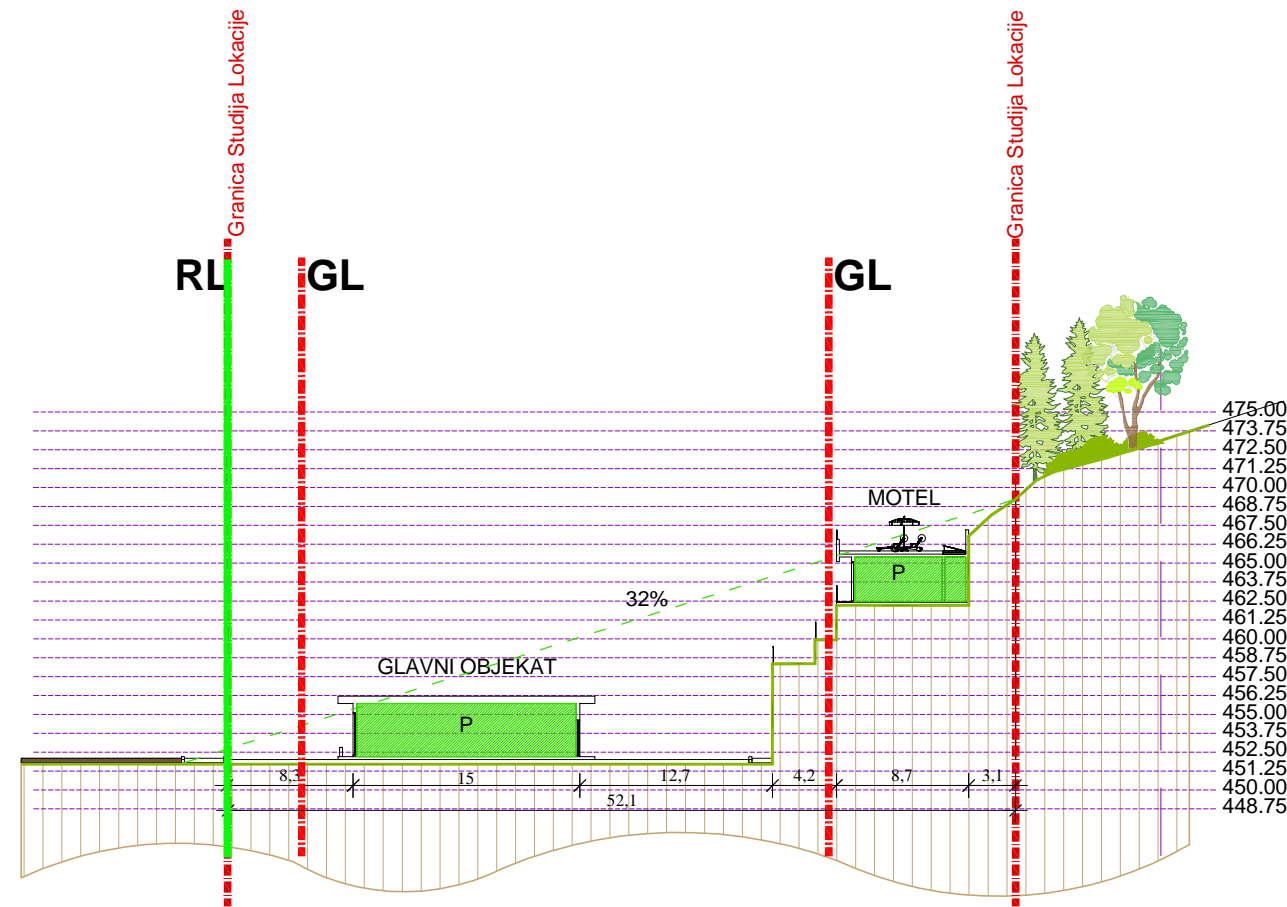
PRESJEK 3-3
