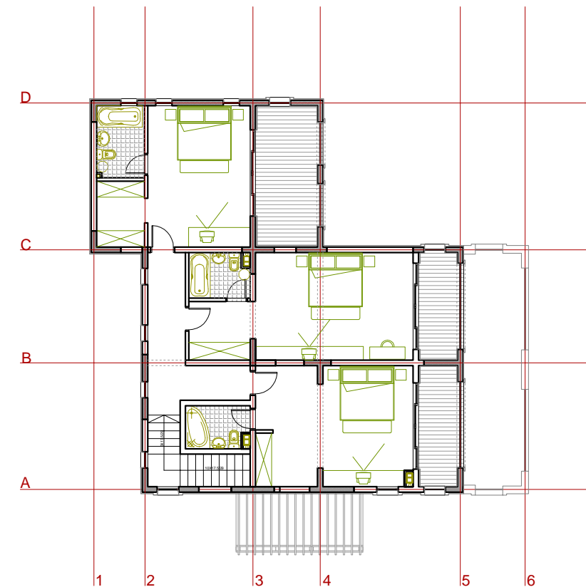
OSNOVA SPRATA
