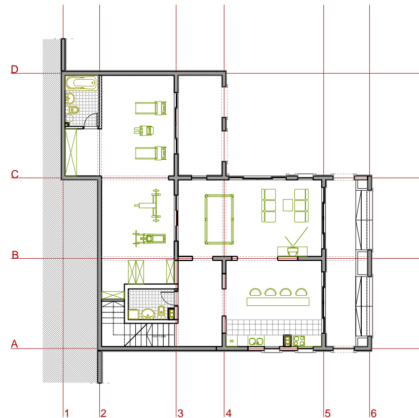
OSNOVA SUTERENA
