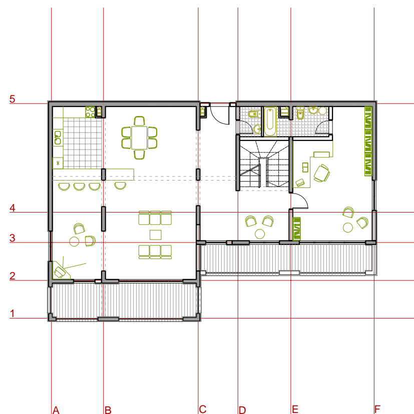
OSNOVA PRIZEMLJA
