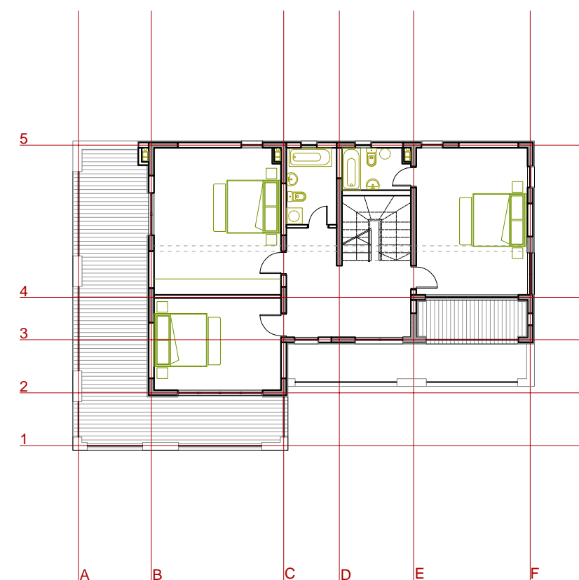
OSNOVA SPRATA
