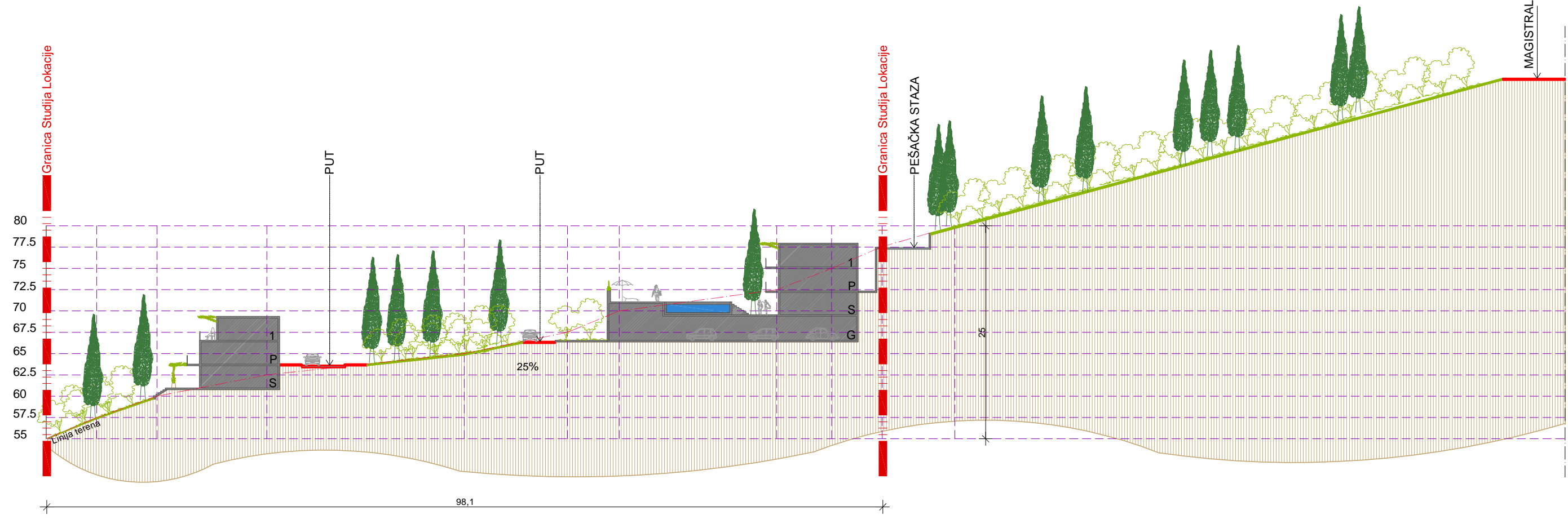
PRESJEK 2-2
