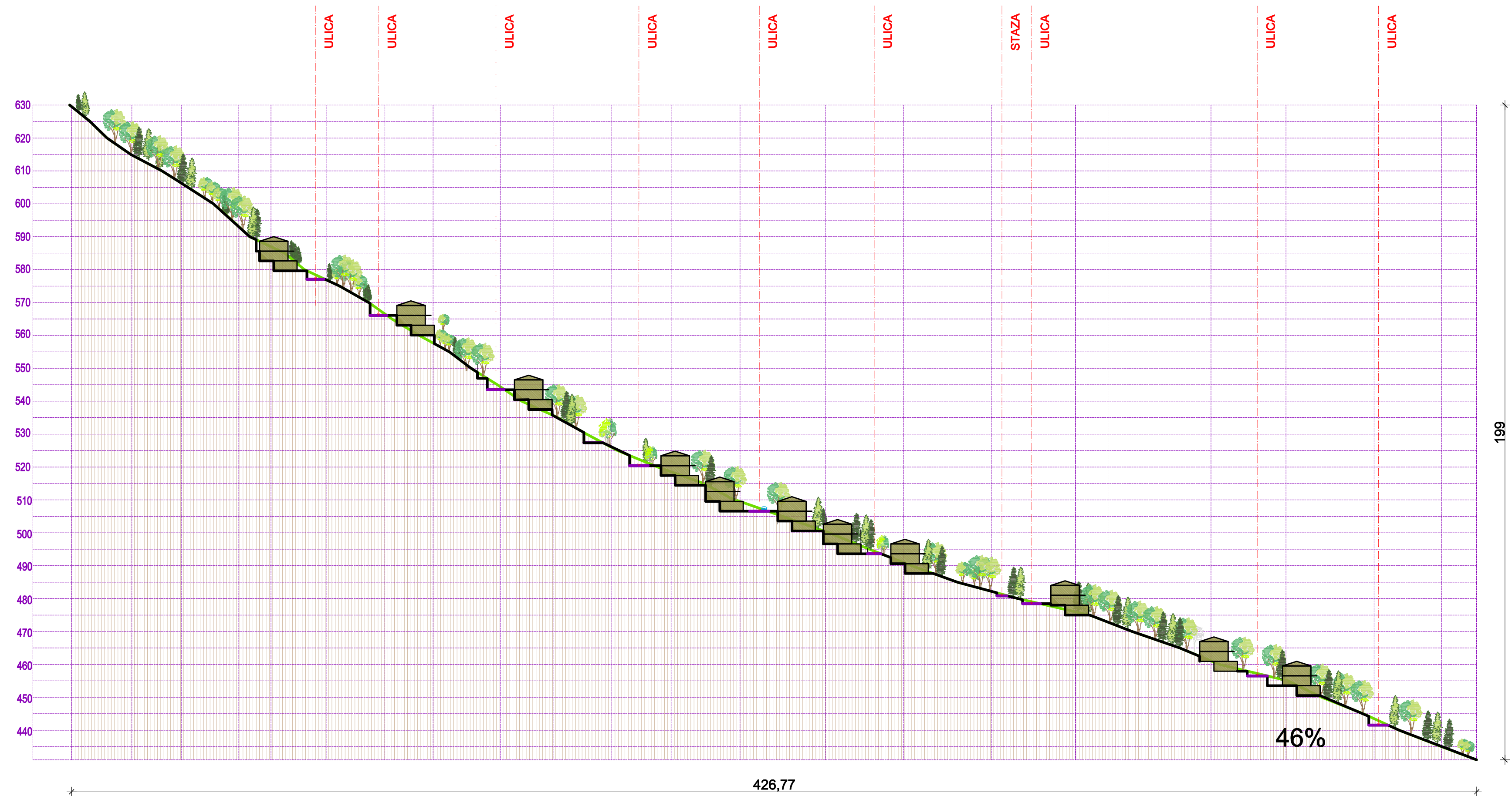
PRESJEK 2-2
