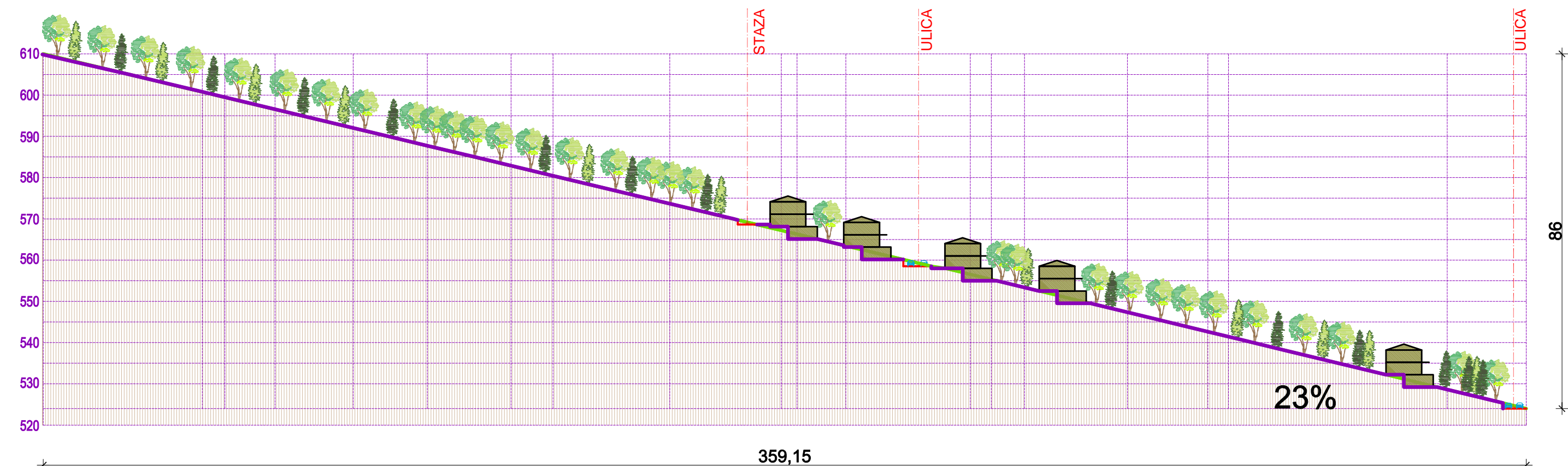
PRESJEK 5-5
