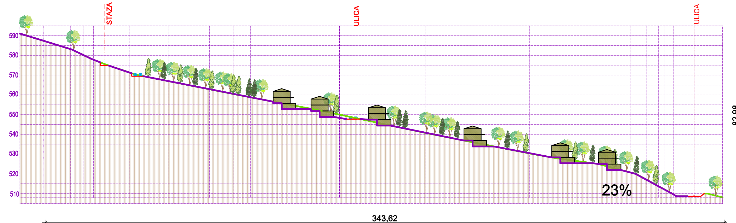
PRESJEK 5-5
