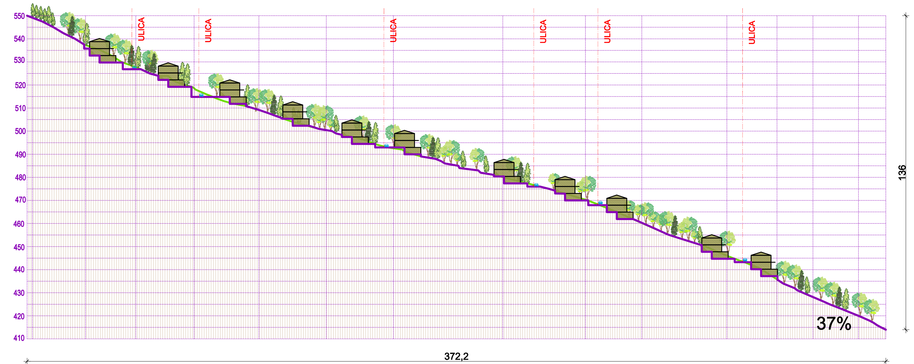
PRESJEK 2-2
