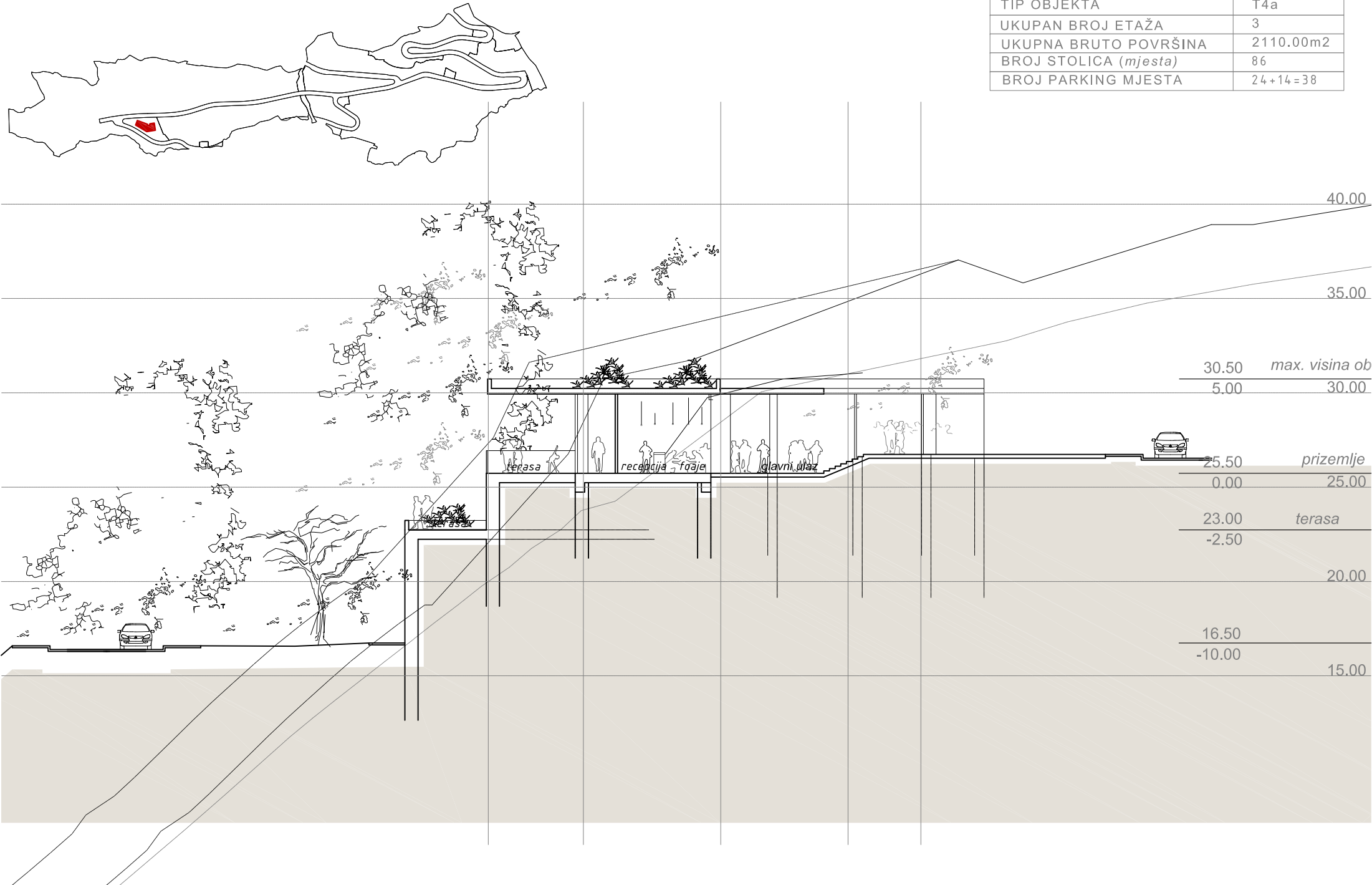
POPREČNI PRESJEK_razmjera 1:250
