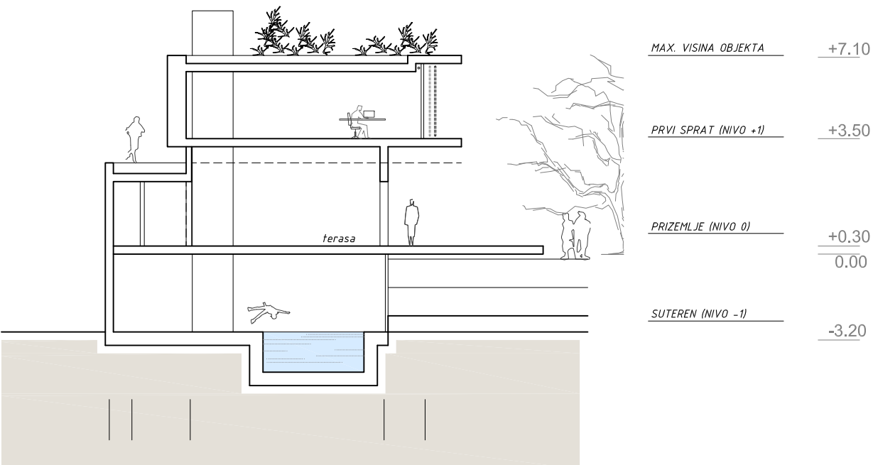
POPREČNI PRESJEK 1
