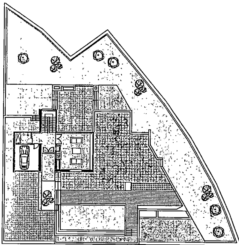
OSNOVA PRIZEMLJA
