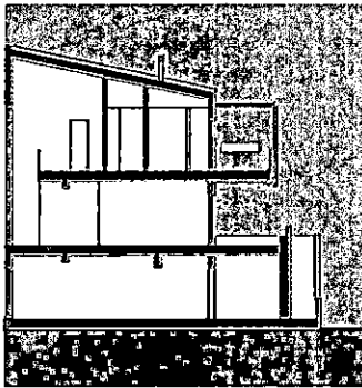
PRESJEK BB'
