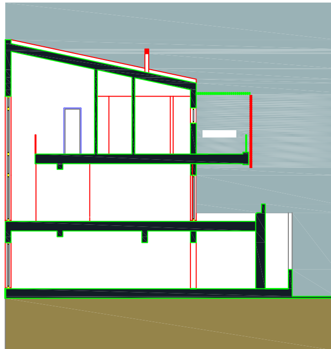
PRESJEK BB'
