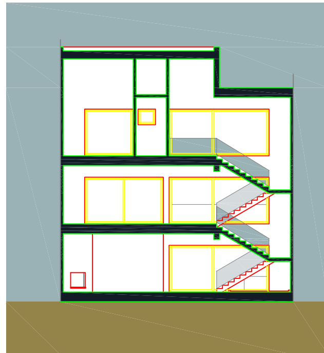
PRESJEK AA'
