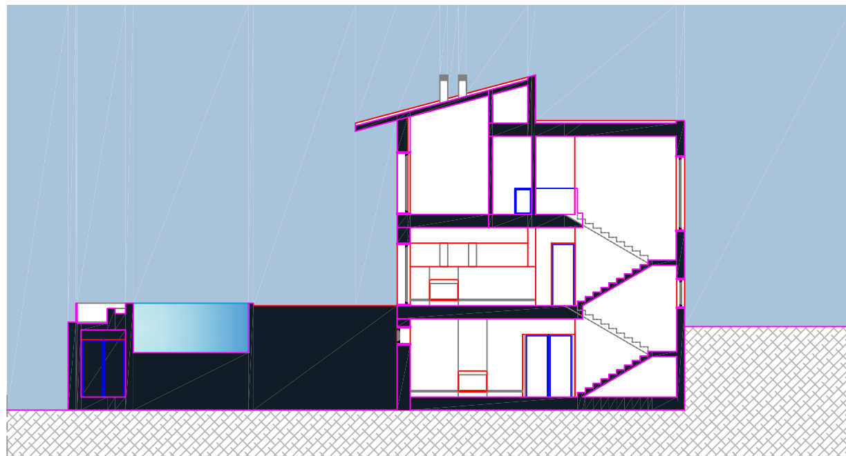
PRESJEK AA'
