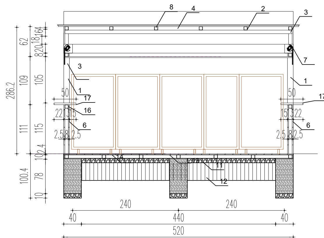
PRESJEK 1-1
