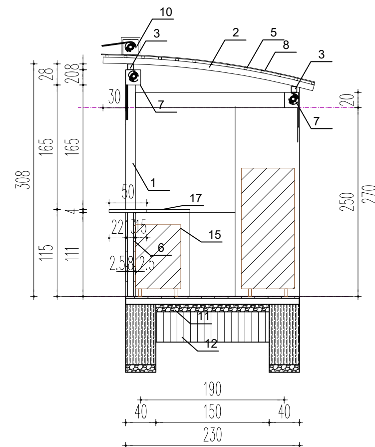
PRESJEK 2-2
