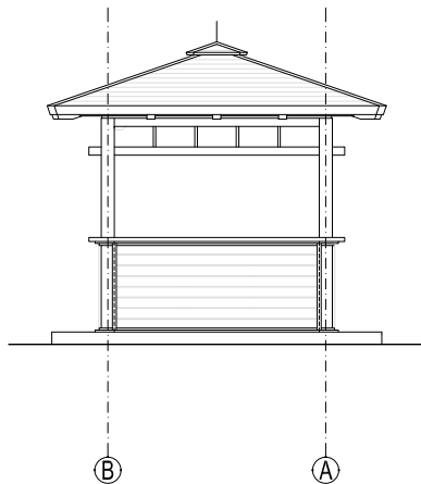
FASADA - ZAPAD
