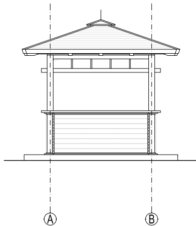
FASADA - ISTOK
