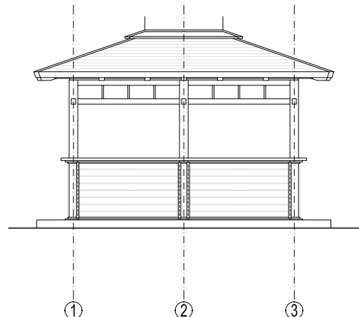
FASADA - JUG
