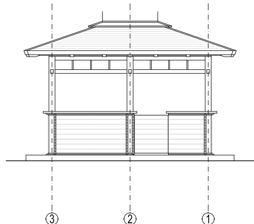
FASADA - SJEVER
