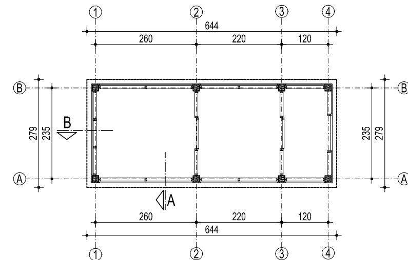
OSNOVA KONSTRUKCIJE BARA
