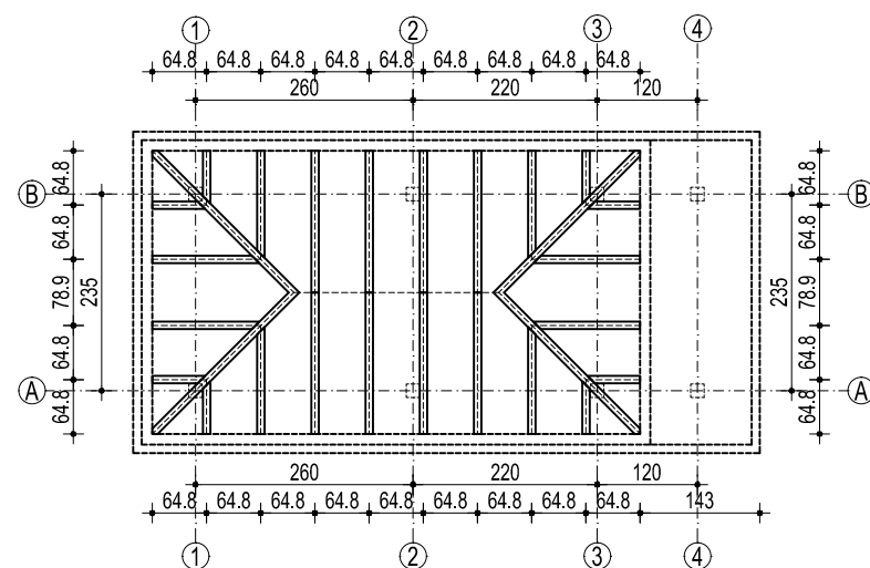
OSNOVA KROVNE KONSTRUKCIJE
