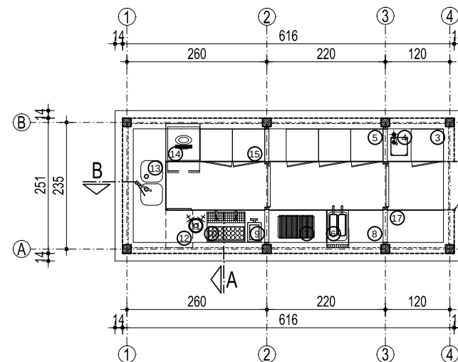
OSNOVA BARA SA OPREMOM
