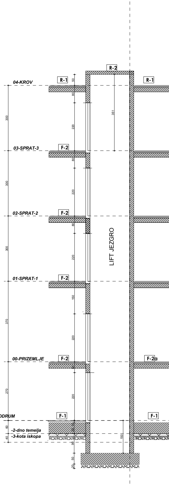
03- PRESJEK A-3
