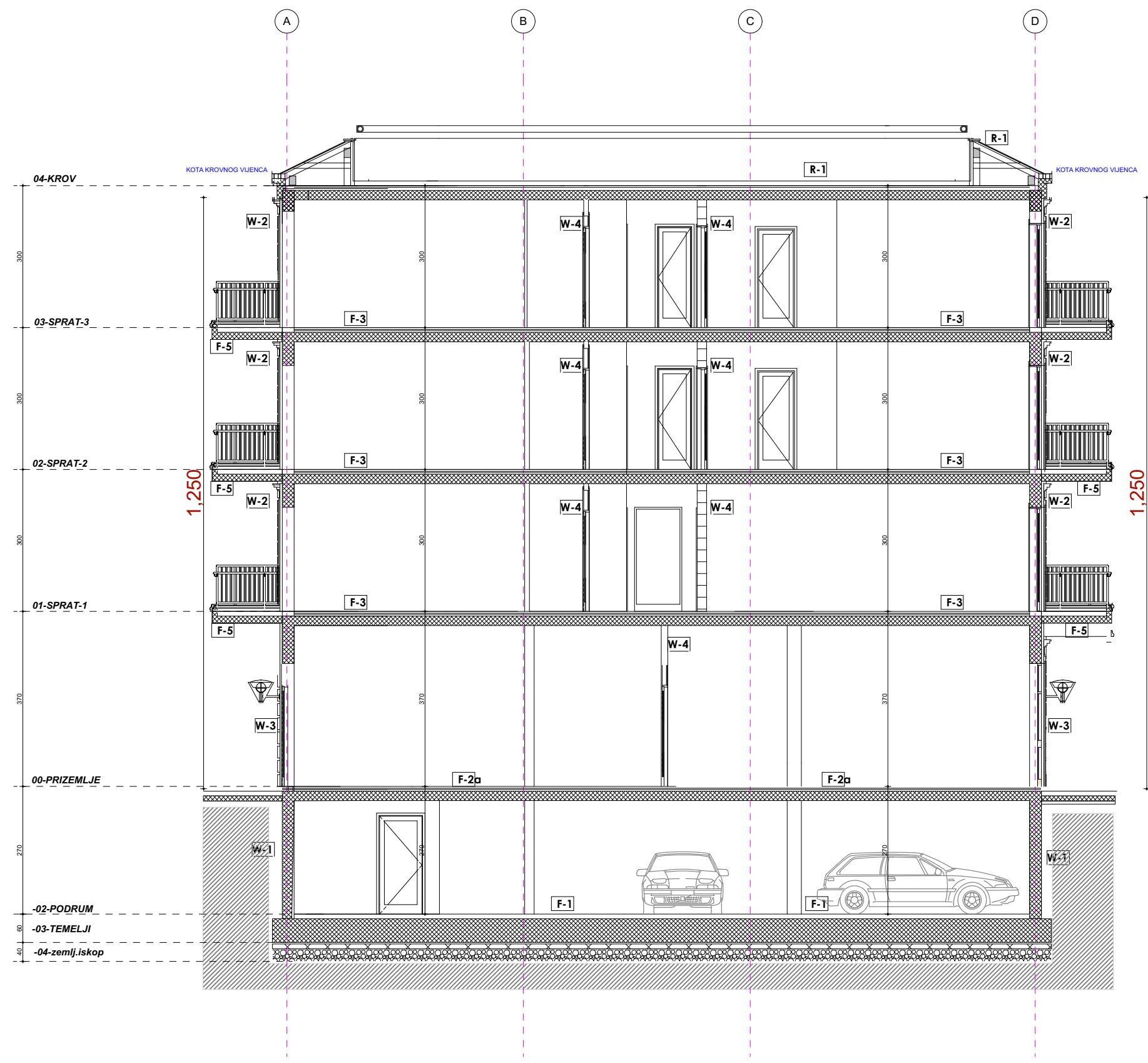
01- PRESJEK A-2
