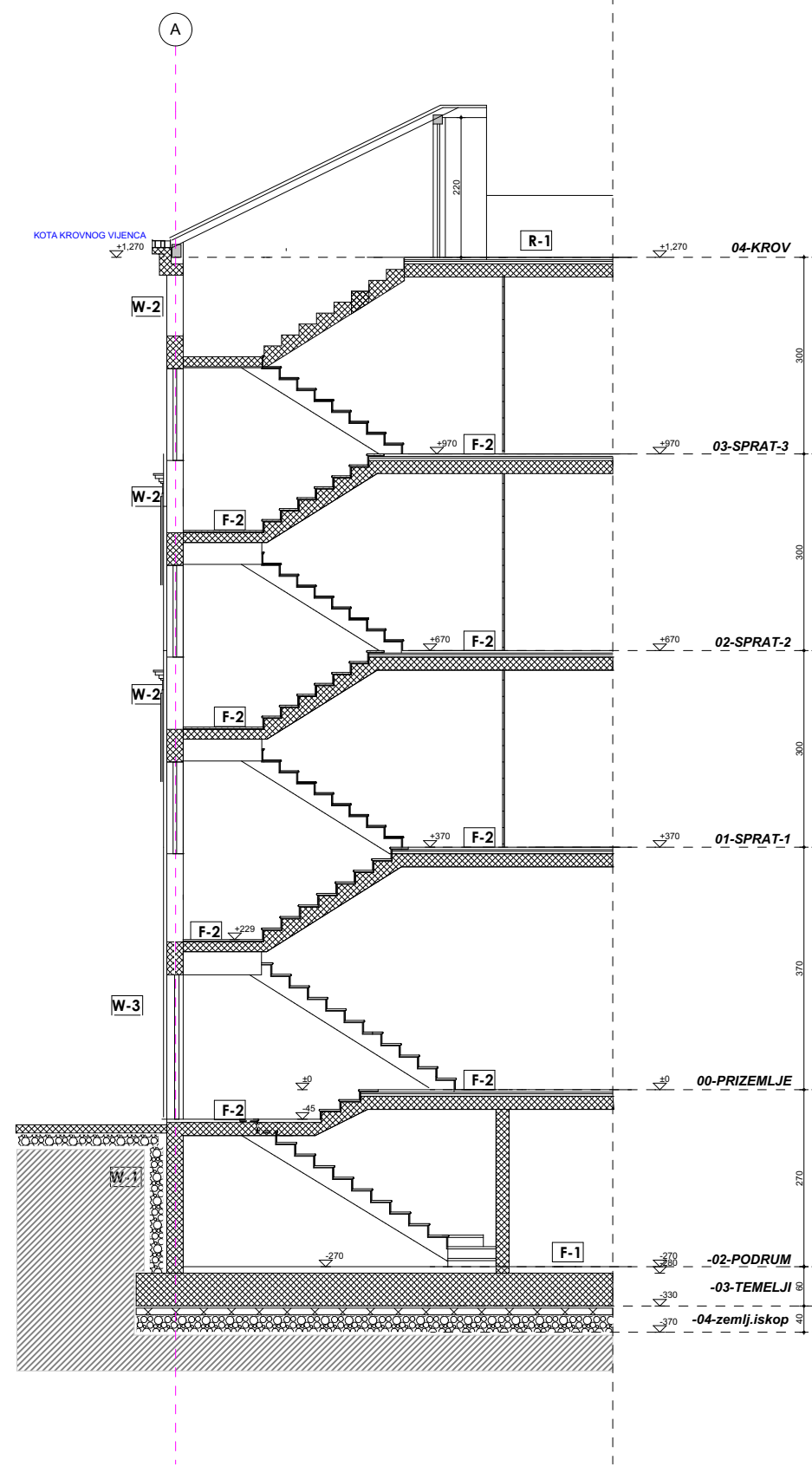
02- PRESJEK A-4
