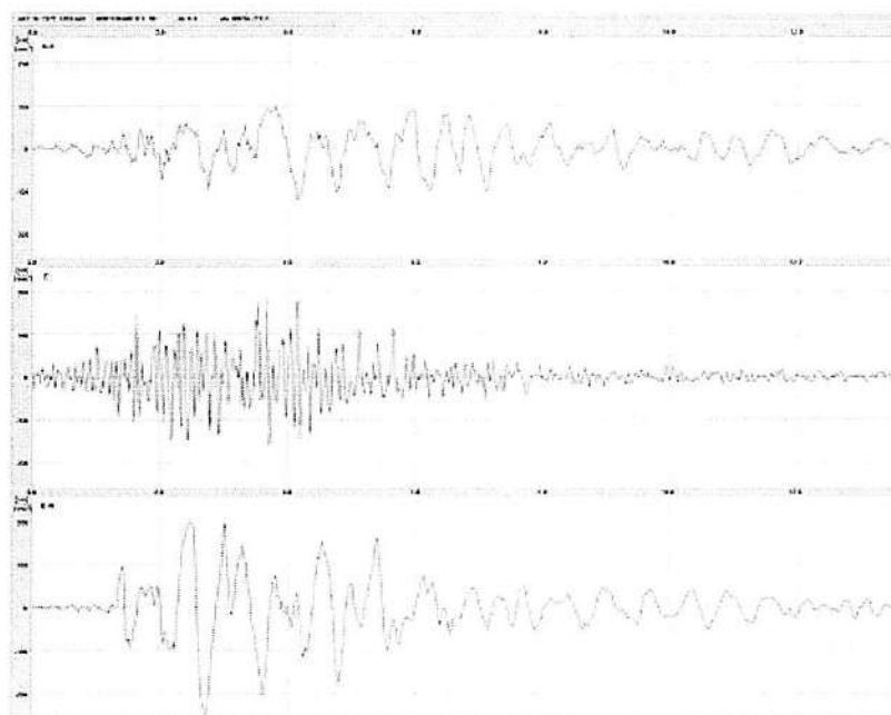
Slika br.18: Karakteristični trokomponentni akcelerogram generisan u najsnažnijem naknadnom zemljotresu u seriji iz 1979. godine u seizmogenoj zoni Budve, 24. maja u 17:23
