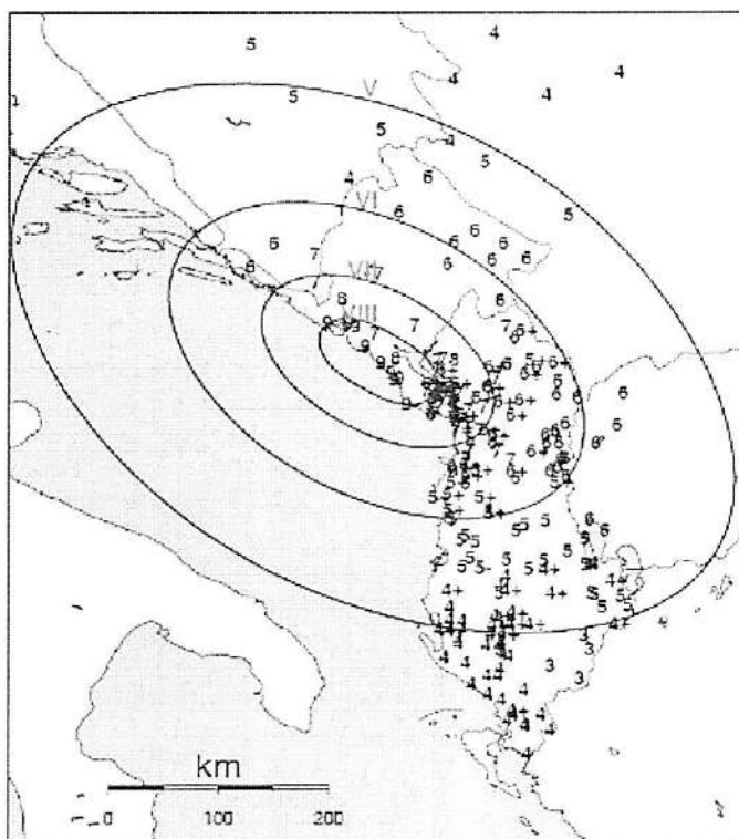
Slika br.20: Izoseiste zemljotresa od 15. Aprila 1979. na crnogorskom primorju, sa magnitudom Mw 7.0 sa izraženom elongacijom u pravcu pružanja Dinarida. Pleistoseista IX (izoseista sa maksimalnim intenzitetom) ovog zemljotresa obuhvatila je praktično cijelo crnogorsko priobalje. Numeričke vrijednosti izražavaju intenzitet ovog zemljotresa, izražen u MCS skali.
