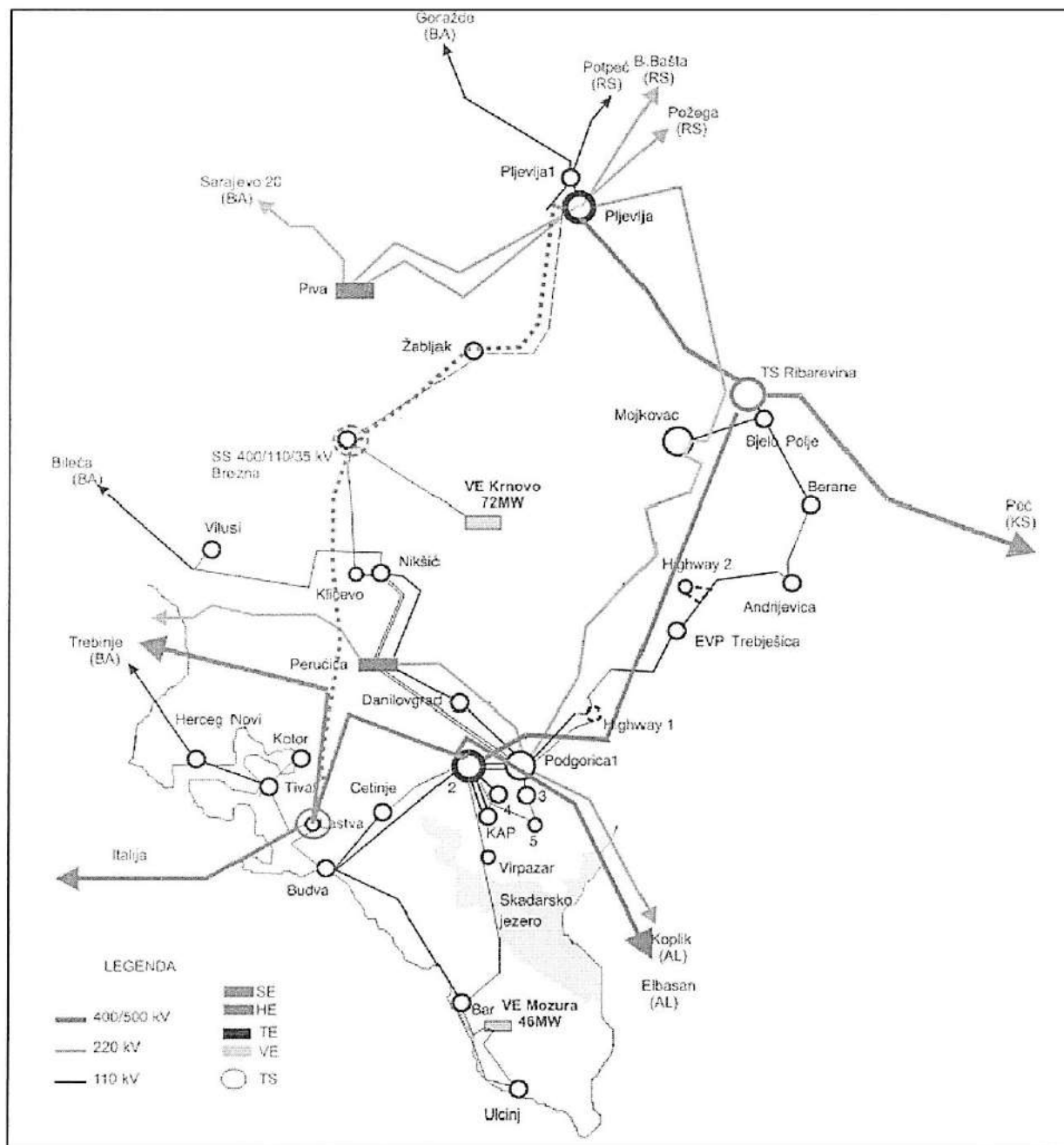
Slika br. 60: Postojeća prenosna mreža – izvor Prostorni plan CG
