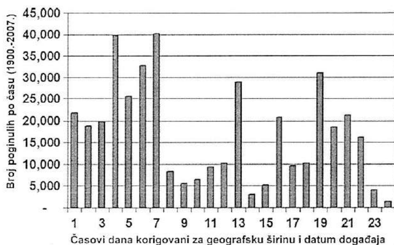
Slika br.63: Ukupan broj poginulih lica na sjevernoj hemisferi, izražen po časovima dana lokalnog vremena, korigovan za dužinu dana i geografsku širinu podatka za period 1900. – 2007. godina (Scawthorn, 2011).
