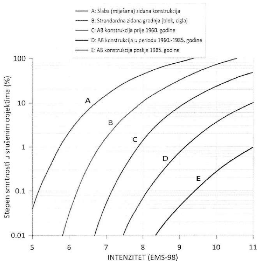
Slika br.65: Stepenn smrtnosti za različite klase povredljivosti degradiranih objekata (A-E) u funkciji makroseizmičke skale intenziteta (EMS-98), Tiedmann (1992).
