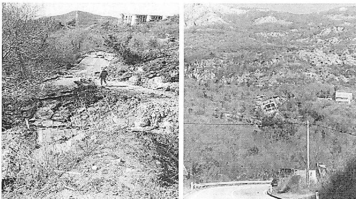
Slika br.14: Klizište Markovići na magistralnom putu Budva - Cetinje
