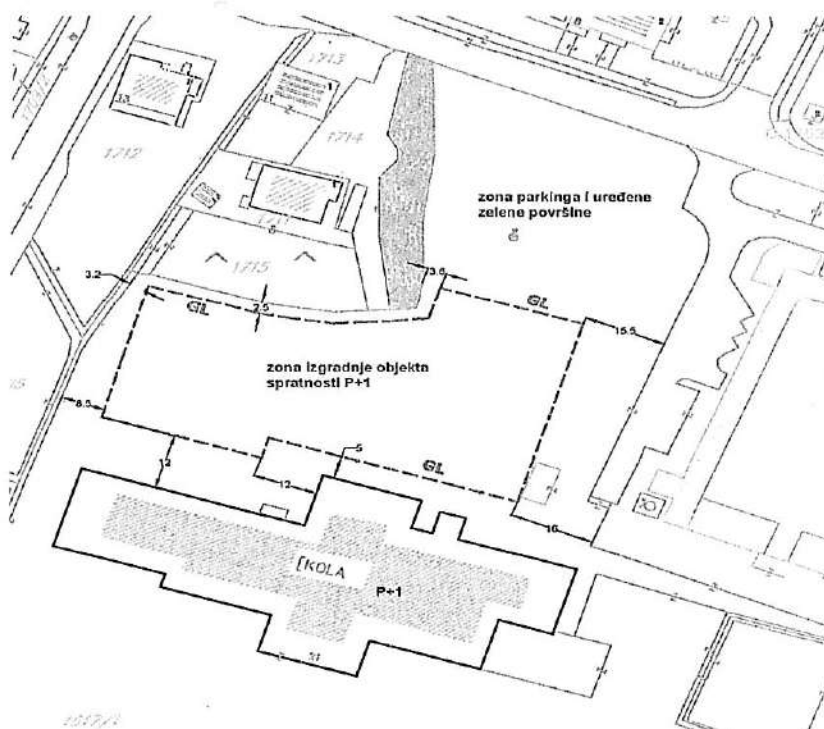
Predlog zone izgradnje sportskog objekta, zone parkinga i uređenih zelenih površine
