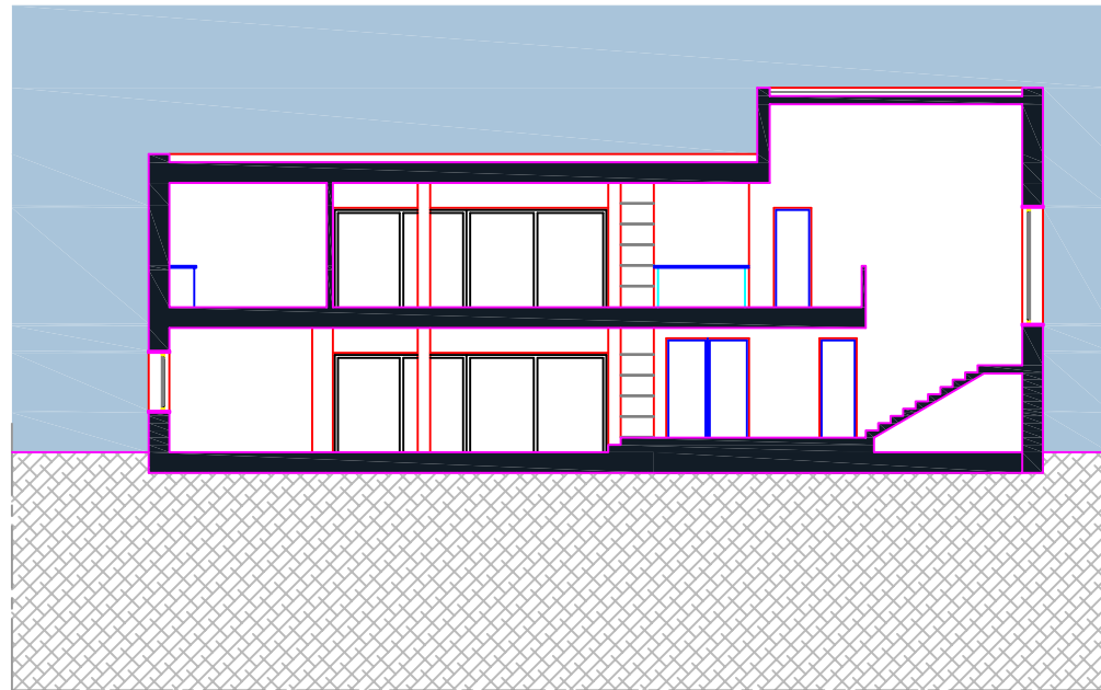
PRESJEK AA'
