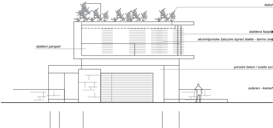
PREDNJI IZGLED
