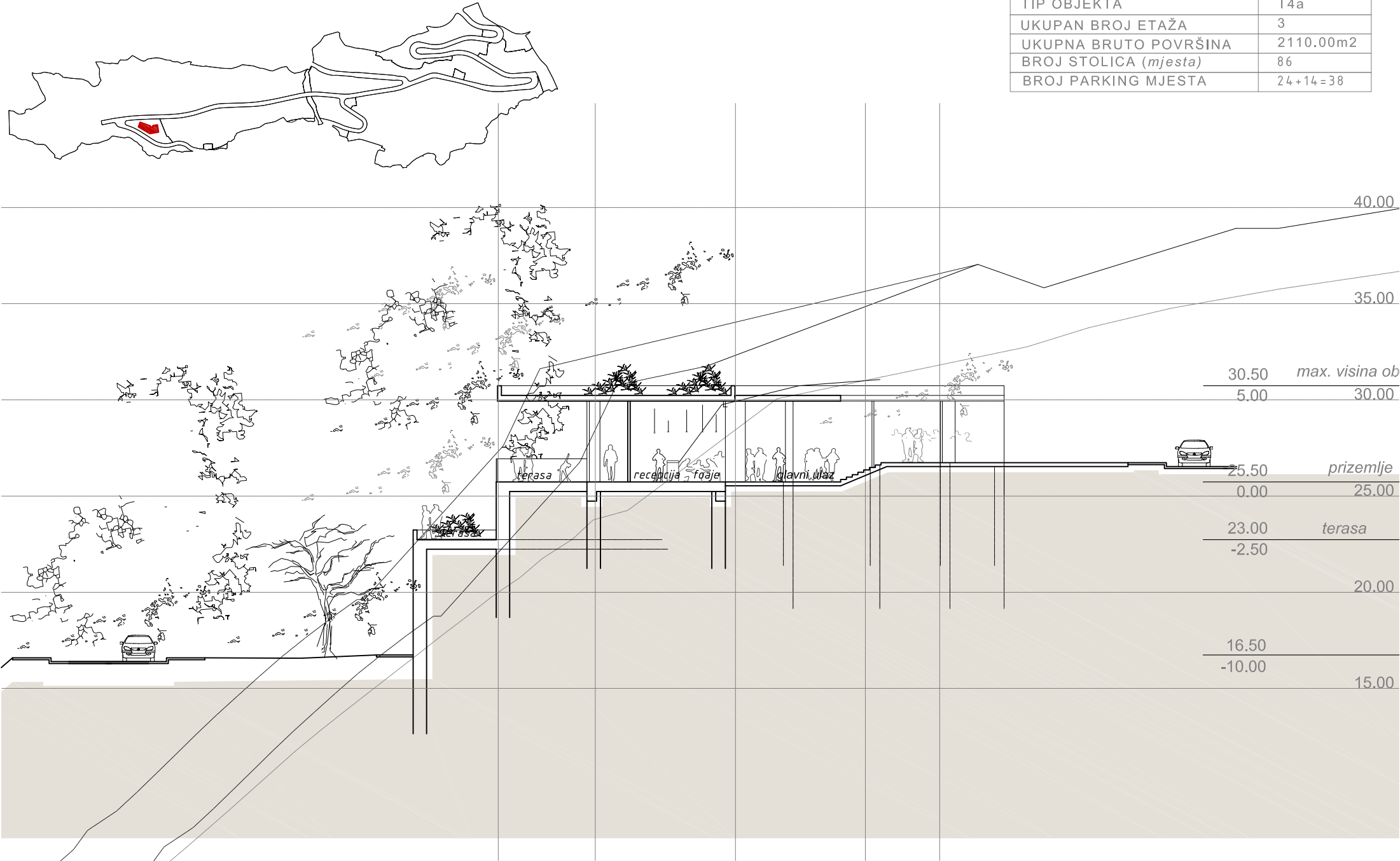
POPREČNI PRESJEK_razmjera 1:250
