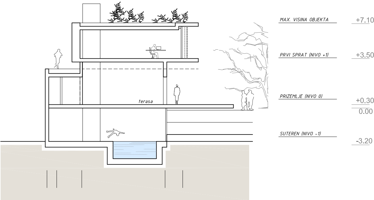
POPREČNI PRESJEK 1
