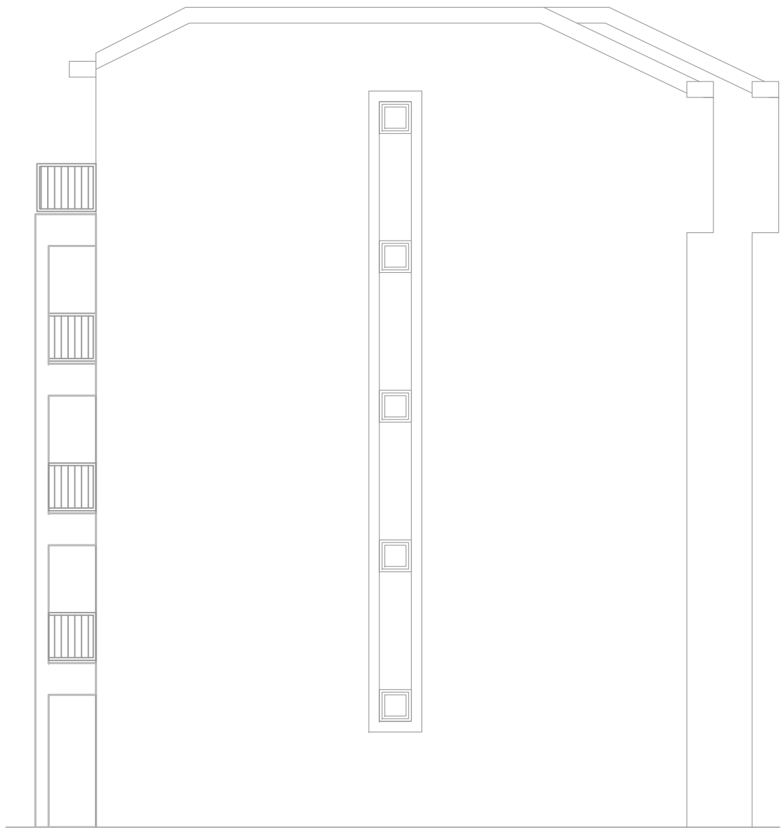
LIJEVA BOČNA FASADA
