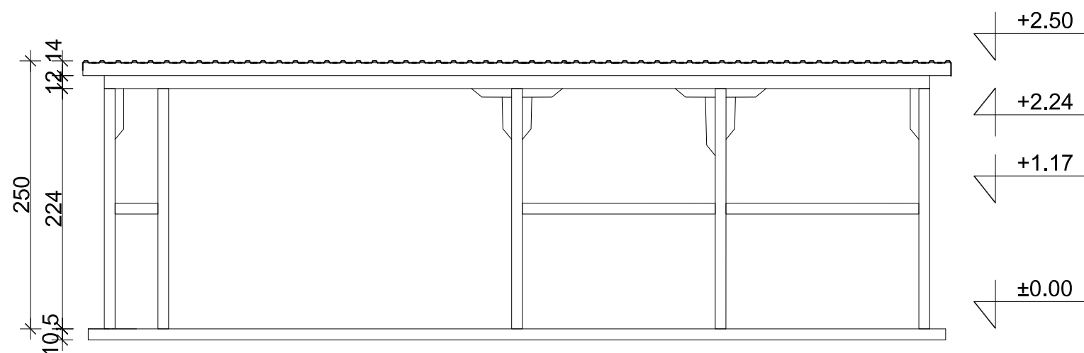
SJEVERO-ZAPADNA FASADA
