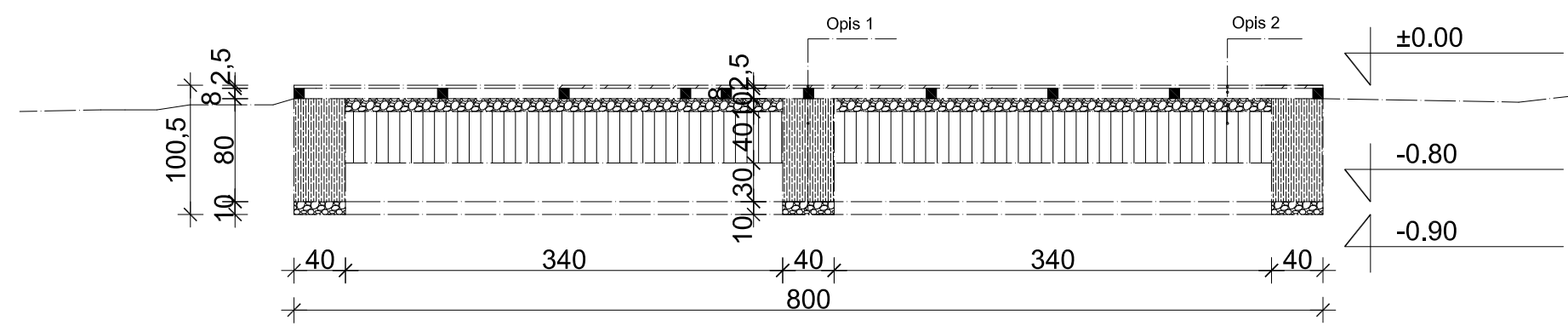
presek 1-1
