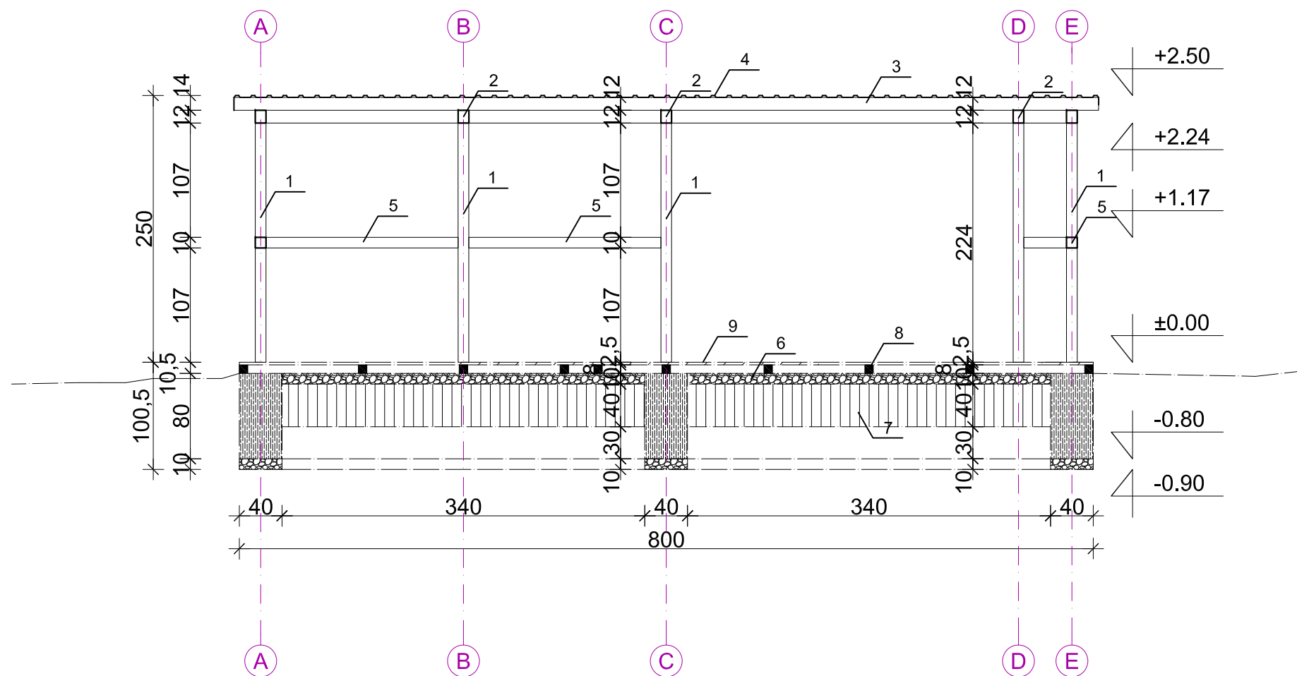
PRESJEK 1-1
