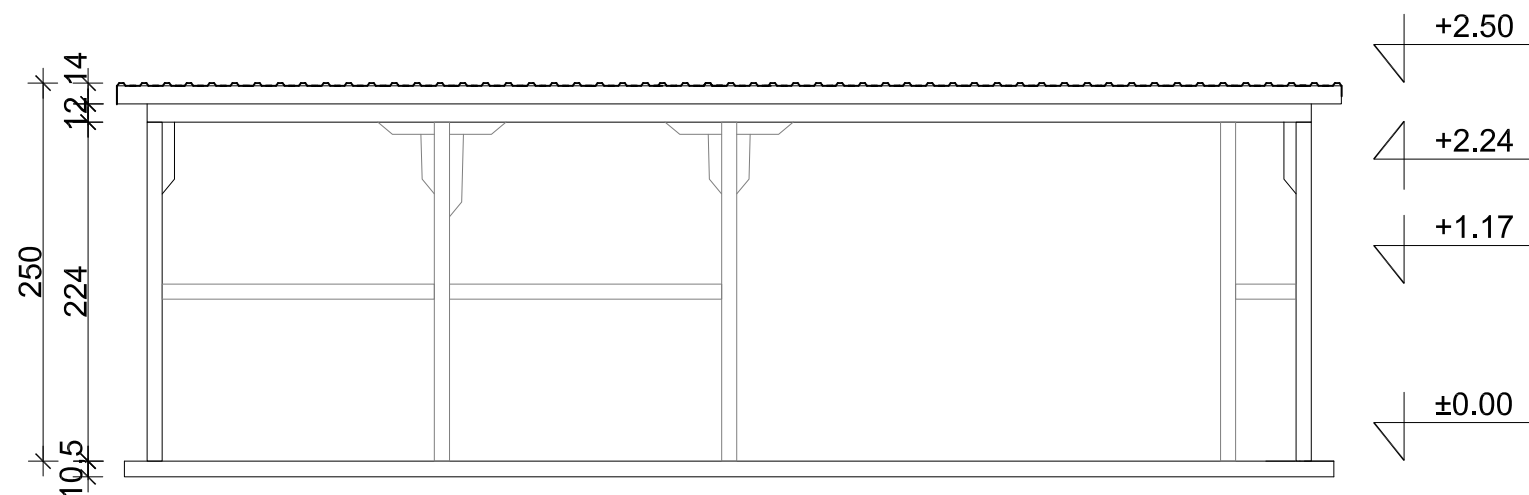
JUGO-ISTOČNA FASADA
