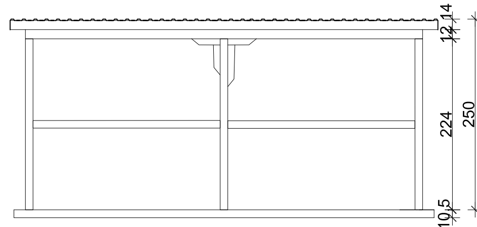
JUGO-ZAPADNA FASADA
