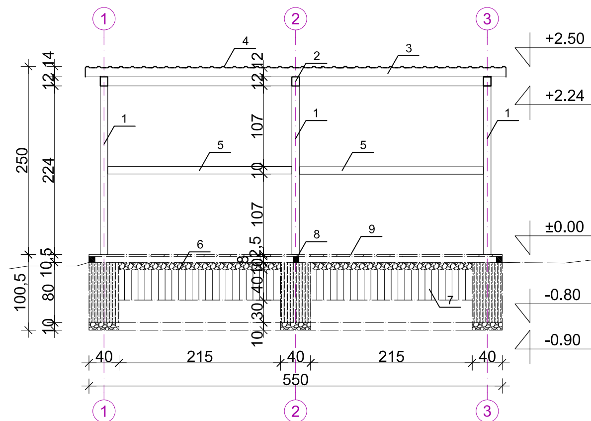
PRESJEK 2-2
