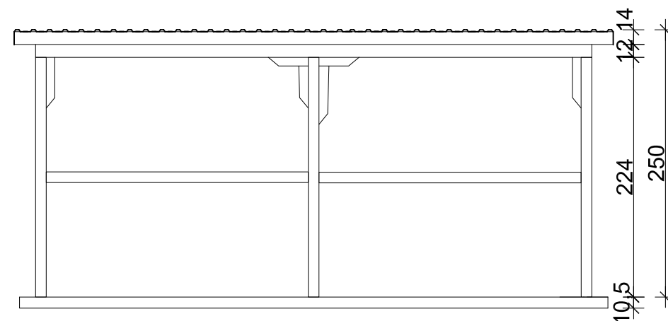
SJEVERO-ISTOČNA FASADA
