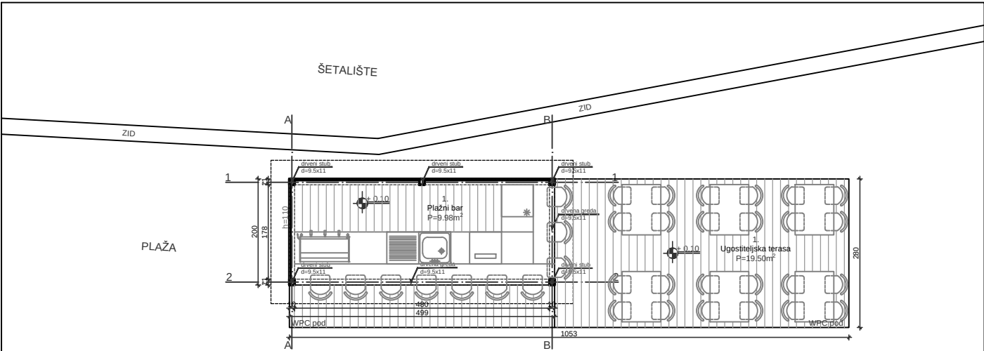
OSNOVA PRIZEMLJA
