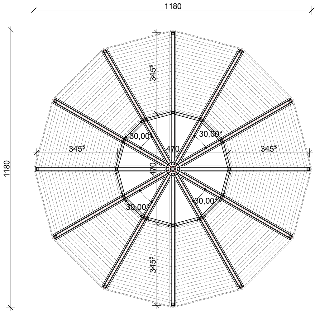
OSNOVA KONSTRUKCIJE
