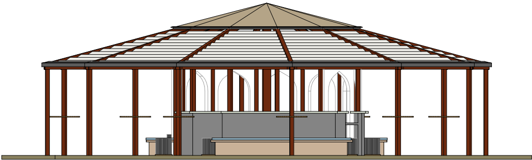
SJEVEROZAPADNA FASADA
