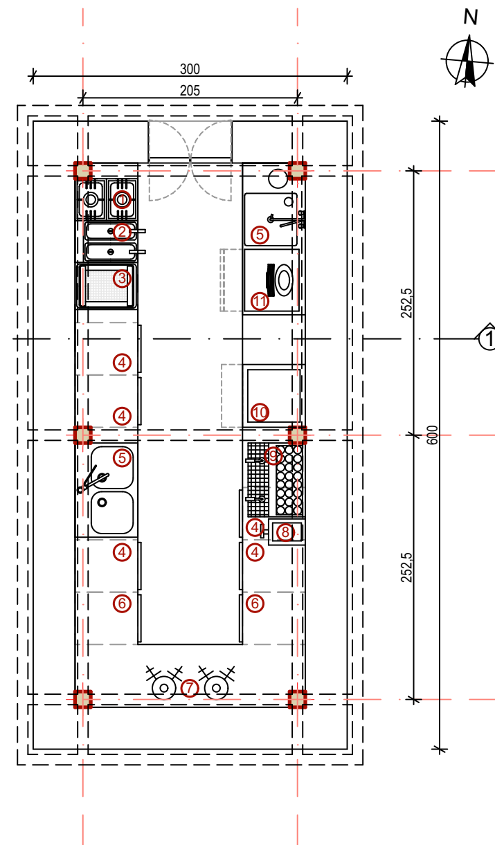
PLAŽNI BAR (OTVORENI ŠANK) BRUTO POVRŠINA 18,00m 2
