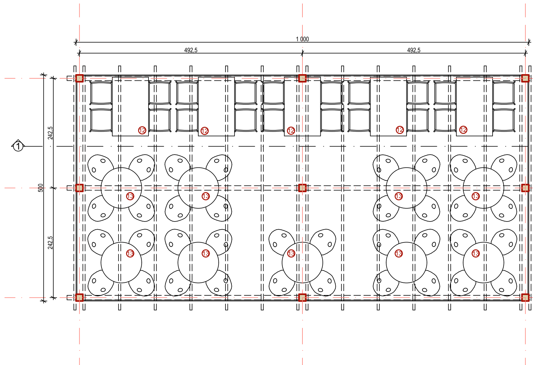
TERASA PLAŽNOG BARA POVRŠINA 50,00m 2
