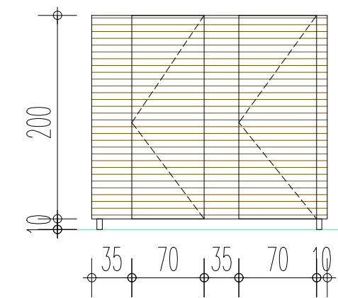
bočni izgled
