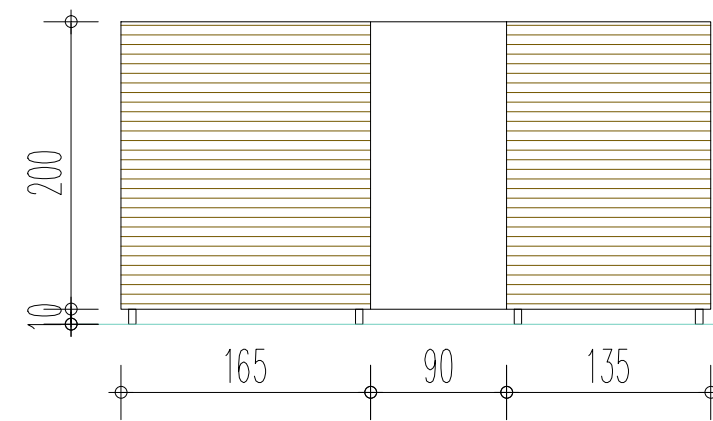
prednji izgled
