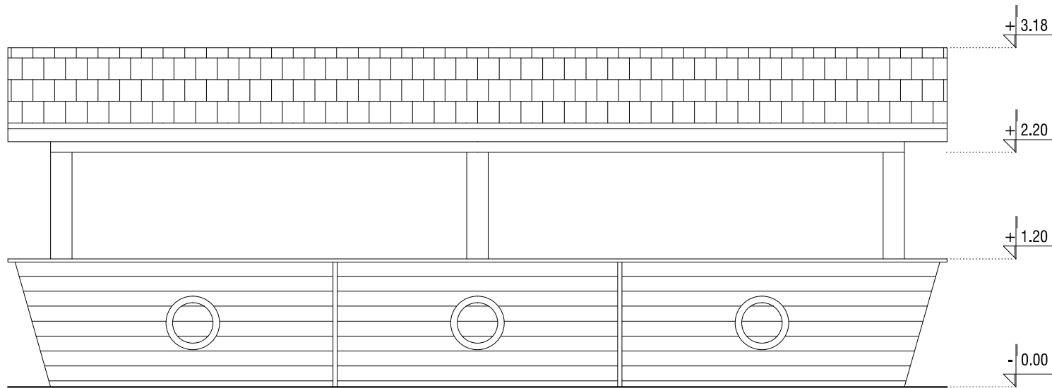
PREDNJI IZGLED
