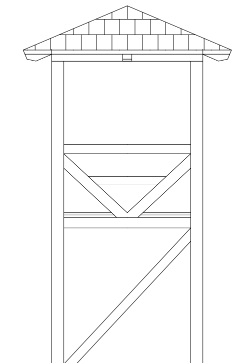
PREDNJI IZGLED
