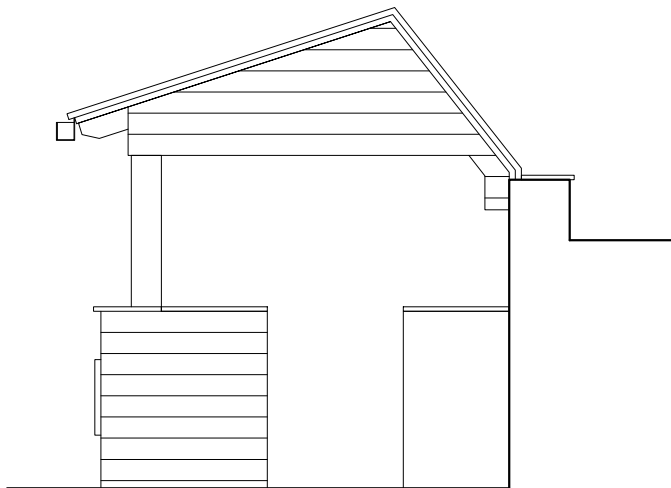
BOČNI IZGLED
