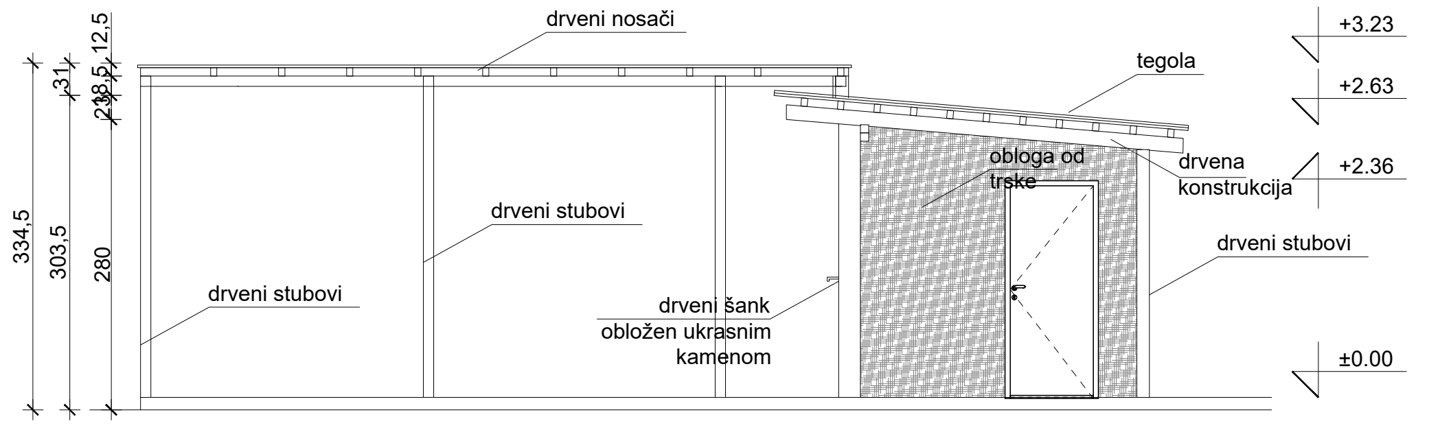
JUGO - ISTOČNA FASADA
