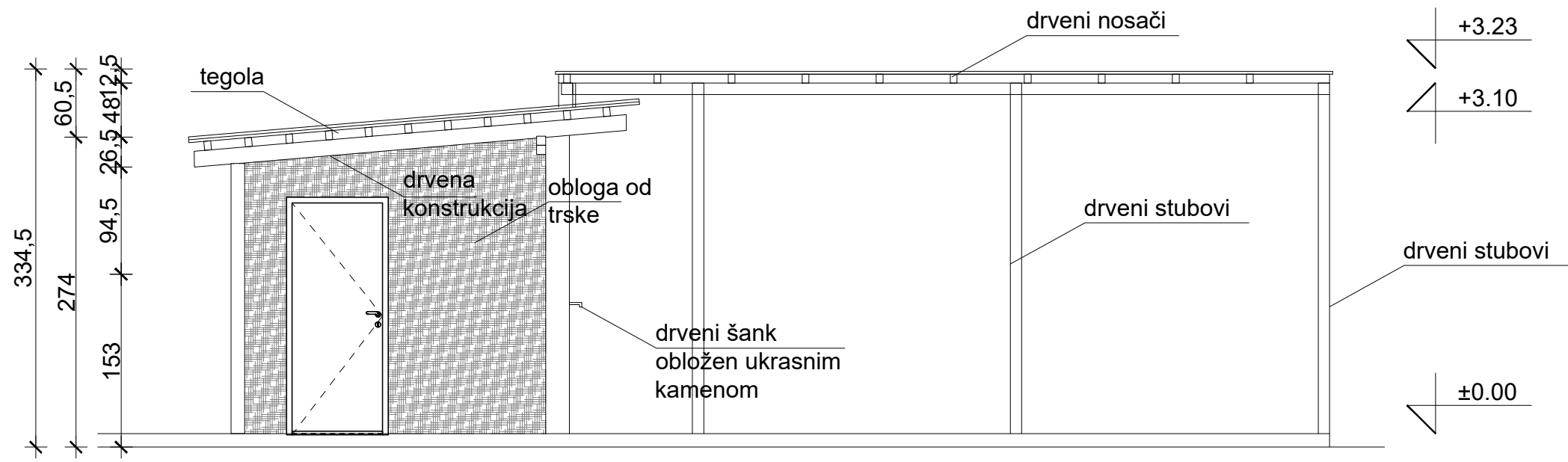
SJEVERO - ZAPADNA FASADA
