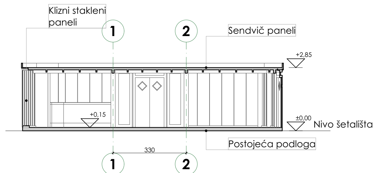
Presek A-A R:100
