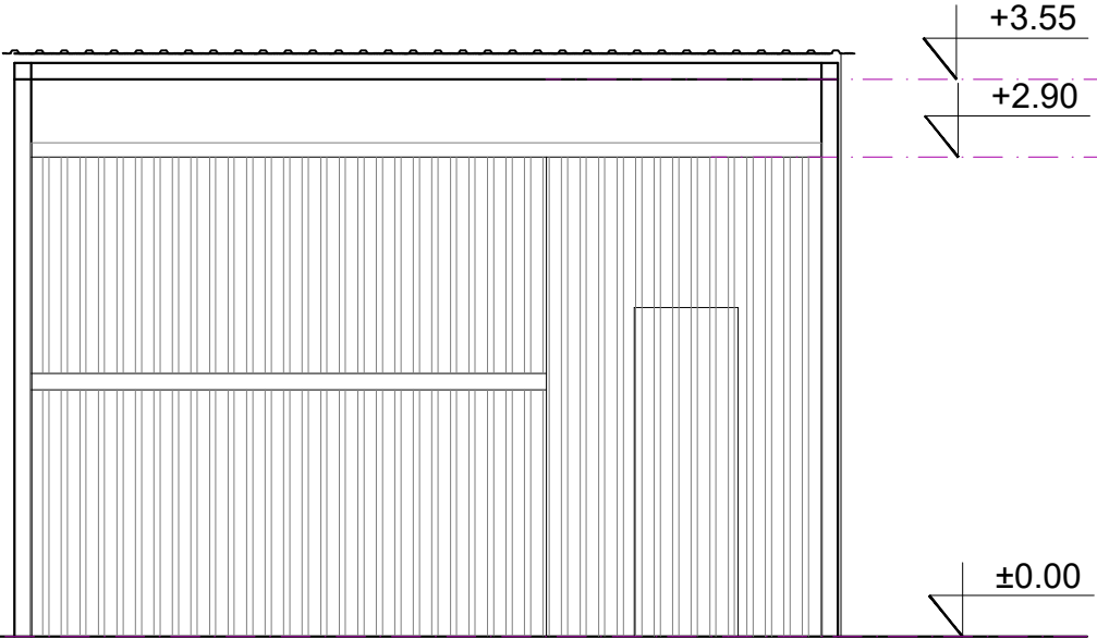
JUŽNA FASADA
