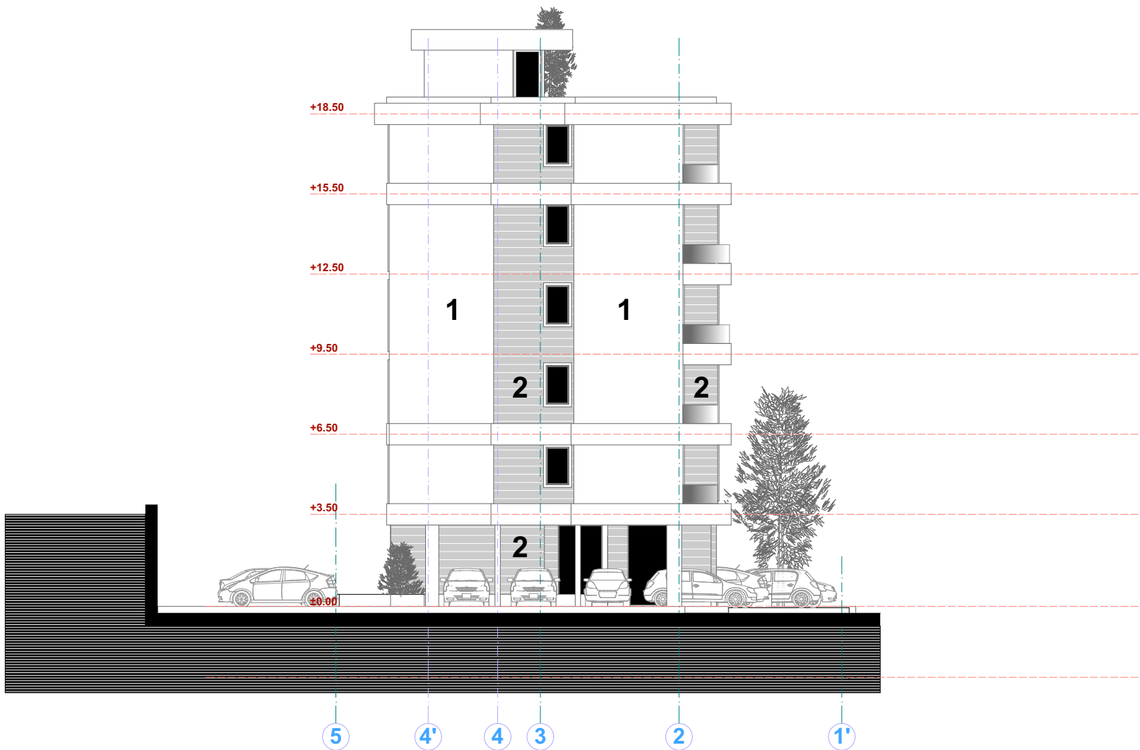
zapadna fasada 1:200
