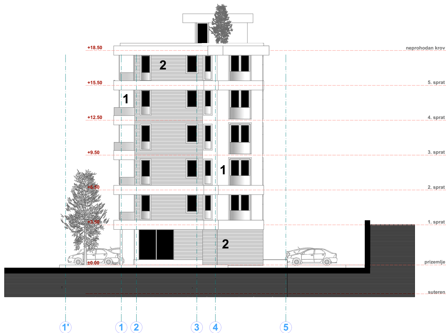
istocna fasada 1:200
