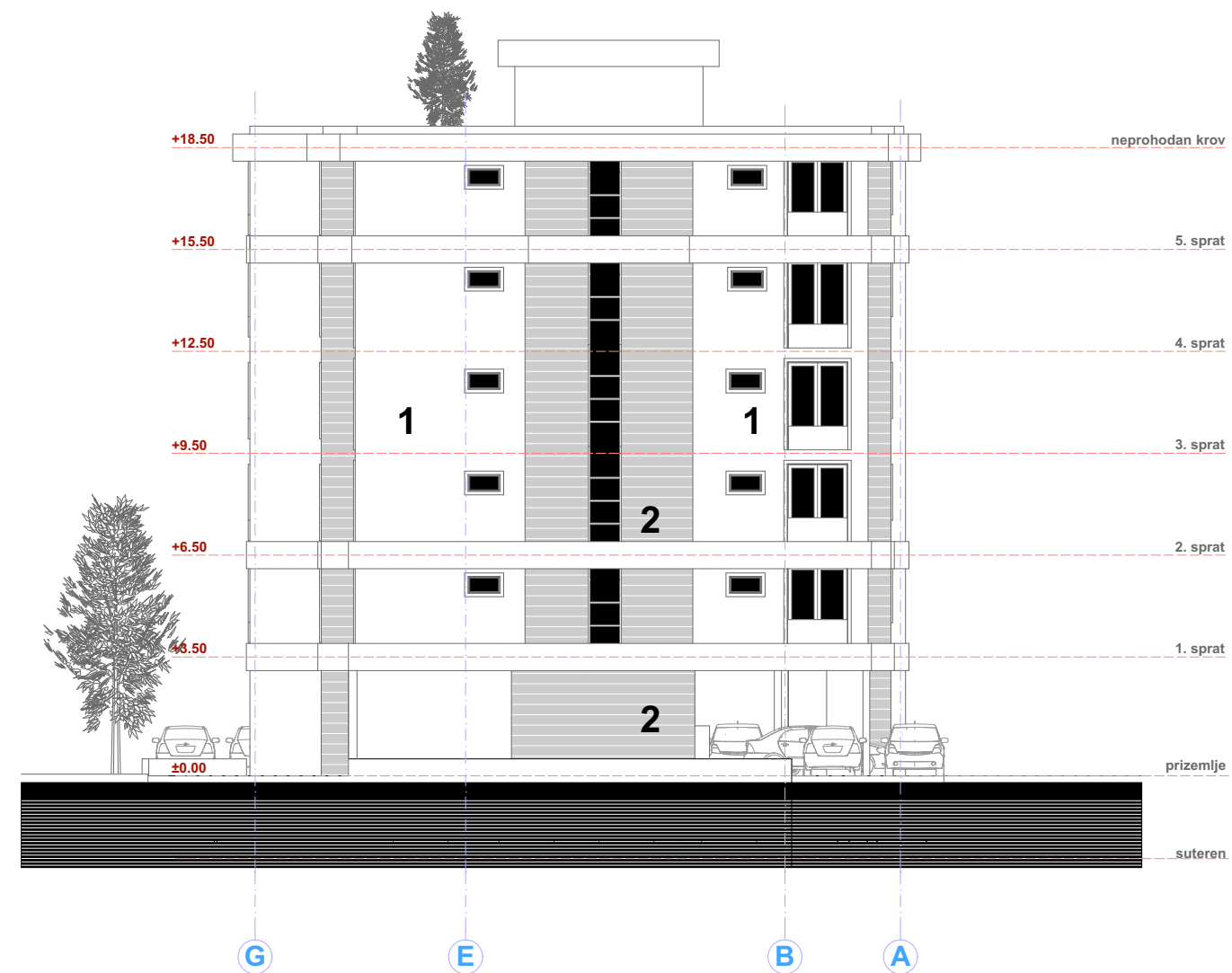
severna fasada 1:200
