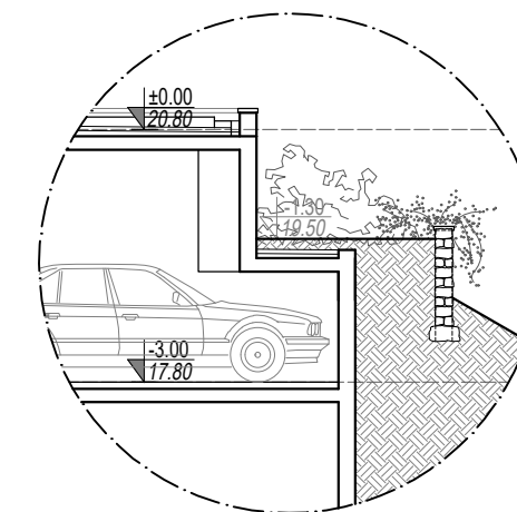
DETALJ: PRESJEK 1-1
